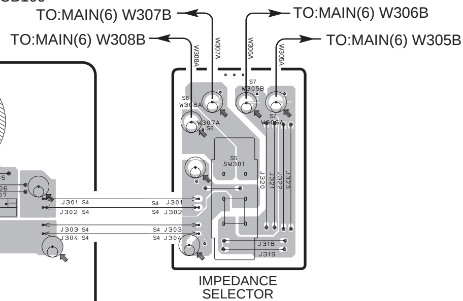
P.C.B MAIN (5)
