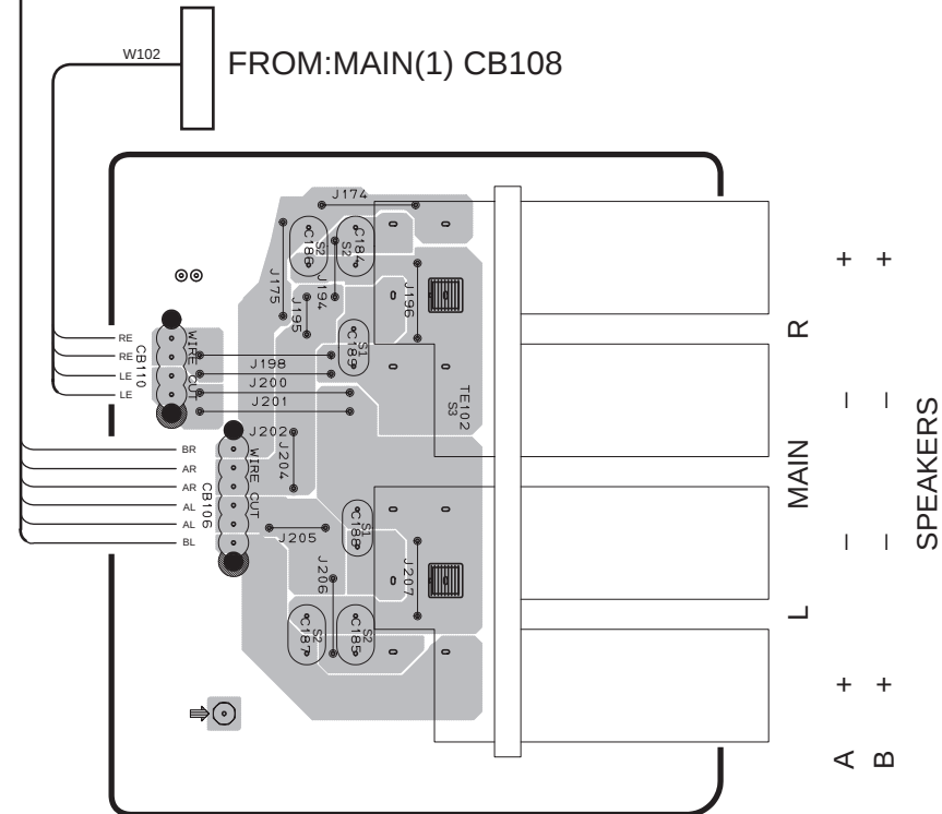
P.C.B MAIN (5)
